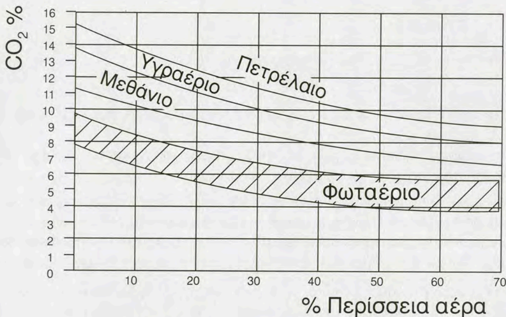
Εικ. 2.4.α Διάγραμμα περίσσειας αέρα
