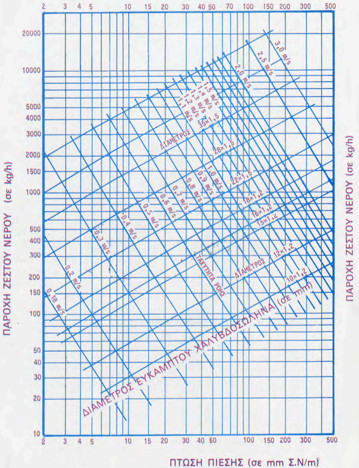
Εικ. 7.2.ζ Χαρακτηριστικά εύκαμπτων χαλυβδοσωλήνων ενός κατασκευαστή
