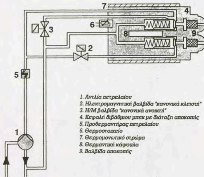
Εικ. 5.1.δ Διβάθμιος καυστήρας διασκορπισμού
