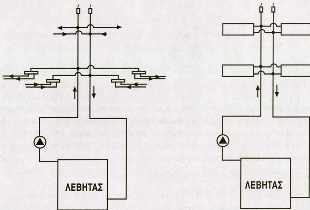
Εικ. 7.1.β Σχηματική παράσταση δικτύου με ένα ζεύγος κατακόρυφων στηλών: αριστερά σε μονοσωλήνιο και δεξιά σε δισωλήνιο σύστημα.
