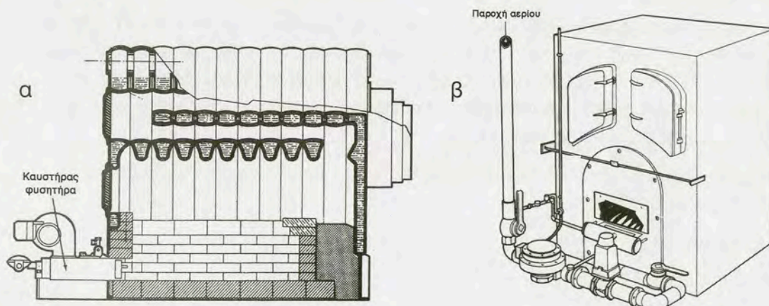
Εικ. 6.2.γ α) πιεστικοί και β) ατμοσφαιρικοί λέβητες αερίου
