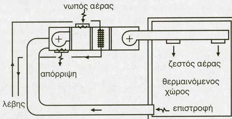
Εικ. 1.1.γ Σχηματική παράσταση εγκατάστασης Κ.Θ. νερού-αέρα
