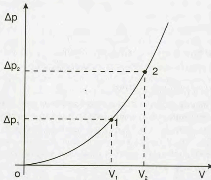
Εικ. 7.2.16 Χαρακτηριστική καμπύλη κυκλώματος
