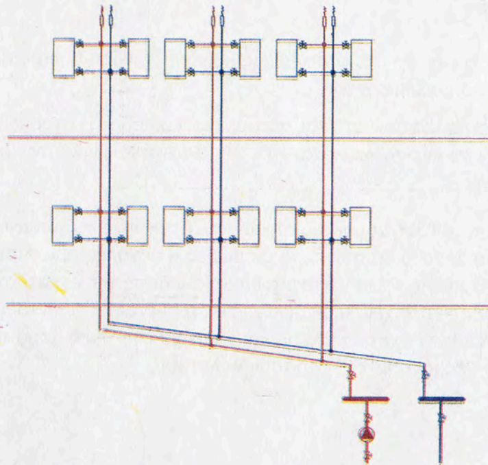
Εικ. 7.2.α Ανάπτυξη δικτύου δισωλήνιου συστήματος με τρία ζεύγη κεντρικών στηλών
