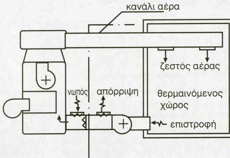
Εικ. 1.1.6 Σχηματική παράσταση εγκατάστασης Κ.Θ.με άμεση θέρμανση του αέρα
