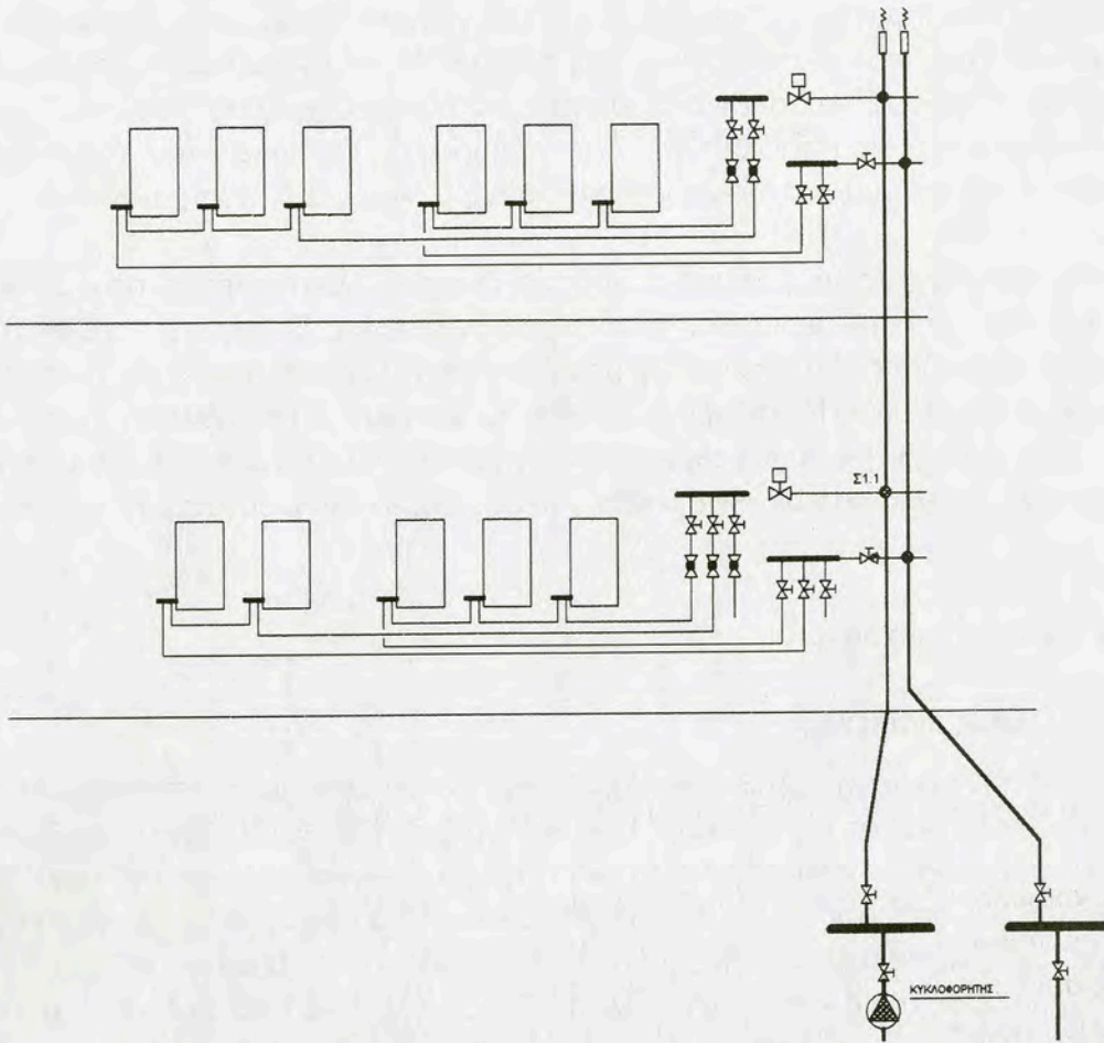
Εικ. 7.2.6 Ανάπτυξη δικτύου μονοσωλήνιου συστήματος με ένα ζεύγος στηλών
