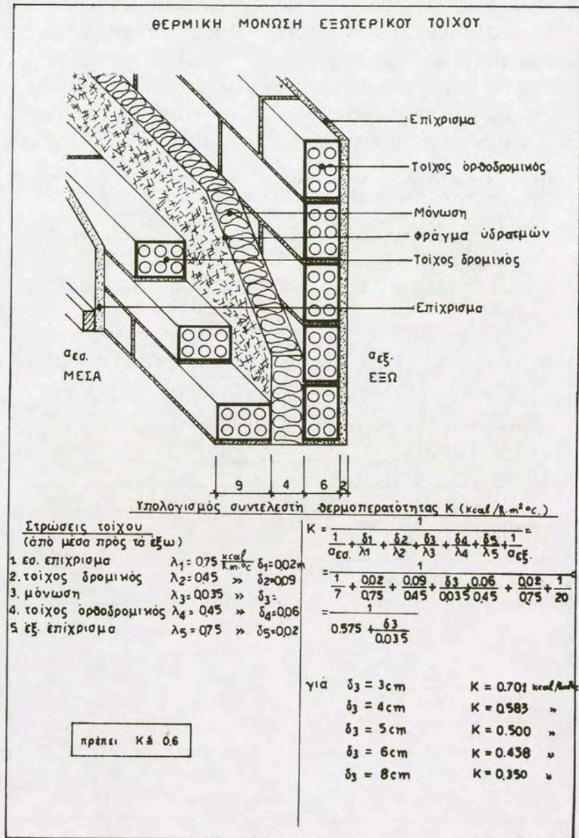
ΕΙΚ. 11.3.6 θερμική μόνωση εξωτερικού τοίχου
