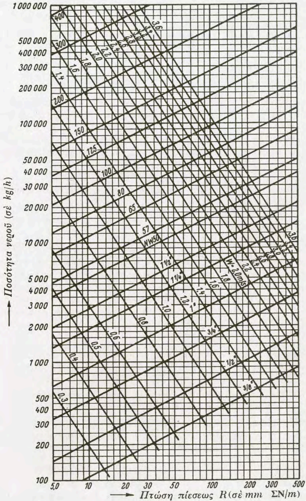
Εικ. 7.2.1 Διάγραμμα χαρακτηριστικών για χαλυβδοσωλήνες
