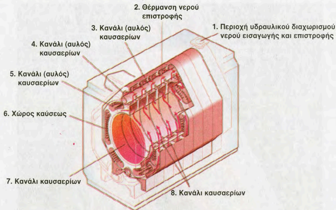
Εικ. 6.2.6 Λέβητας με είσοδο-έξοδο νερού στο πάνω μέρος
