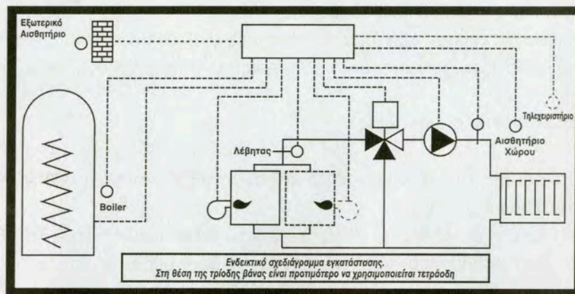
Εικ. 10.2δ Κέντρο αυτοματισμών
