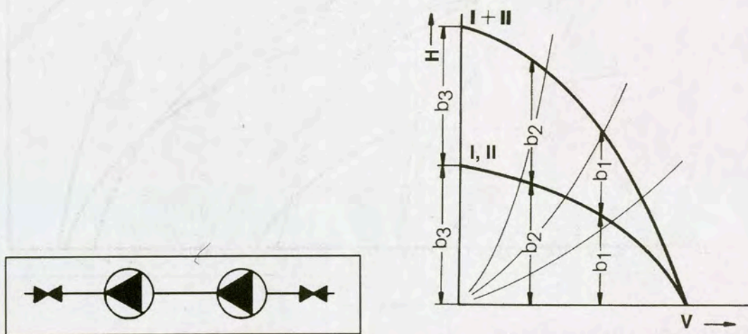
Εικ. 8.3.ε Σύνδεση κυκλοφορητών σε σειρά
