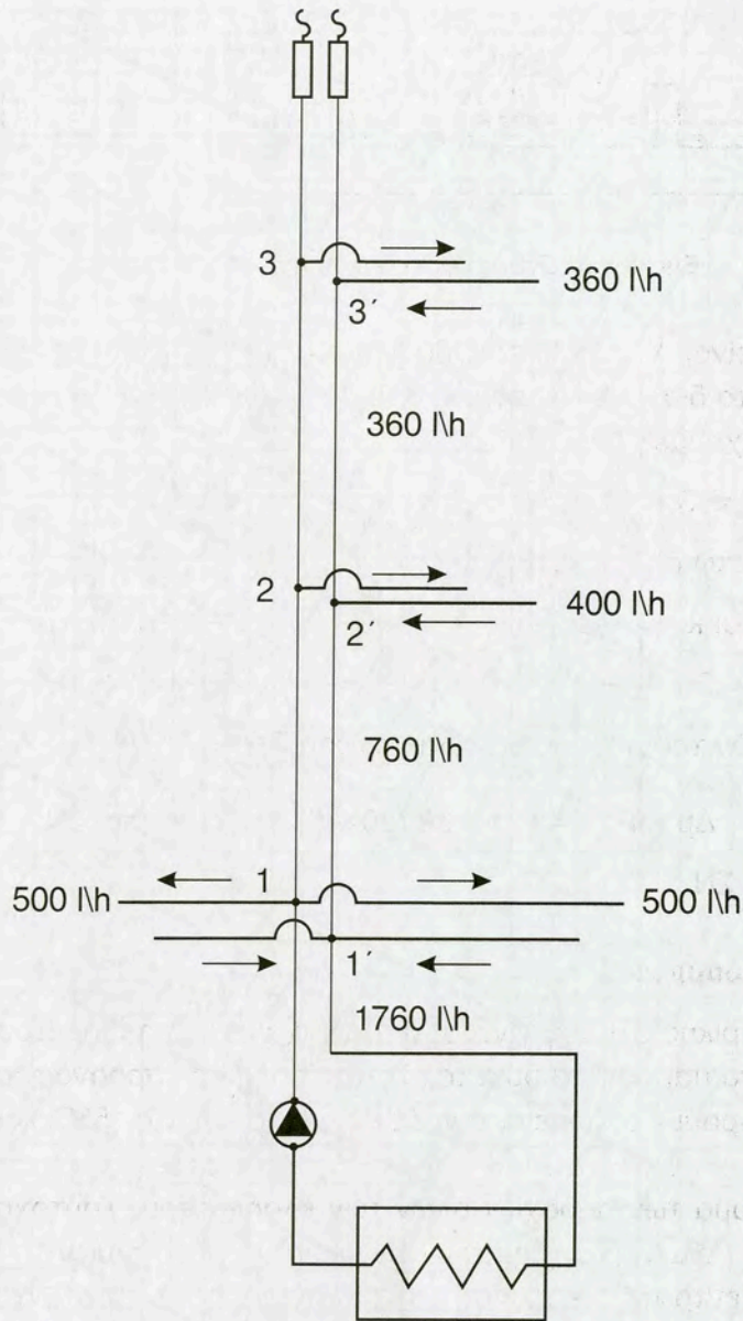
Εικ. 7.2.θ Σχηματική παράσταση κατακόρυφης στήλης του παραδείγματος
